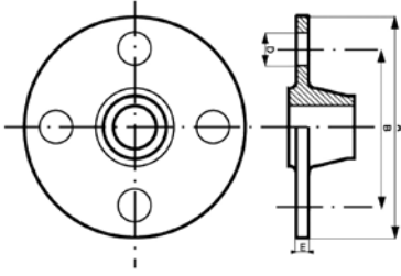
Bride à collerette PN10/16 - 16 type 11B
